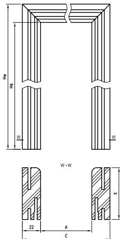
Wymiary paneli poszerzających OR - ościeżnice regulowane do drzwi przylgowych
