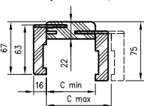
Przekrój TUN z ką. T63
