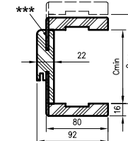
przekrój stojaka
